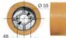
Pogumované kolečko 120x60mm, 45 SHORE Obj.č. 58005 - 490 Kč
