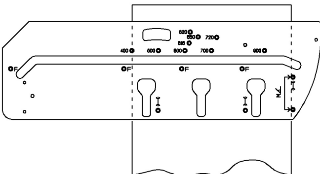
OBRÁZEK C SAMIČÍ SPOJ - LÍCOVÁ STRANA DESKY DOLŮ
