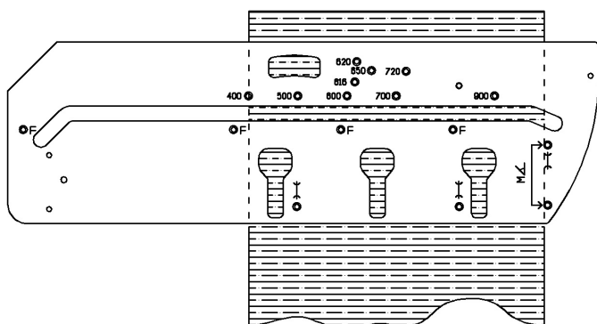
OBRÁZEK C SAMČÍ SPOJ - LÍCOVÁ STRANA DESKY NAHORU
