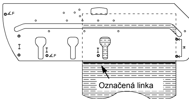
OBRÁZEK B SAMIČÍ SPOJ
