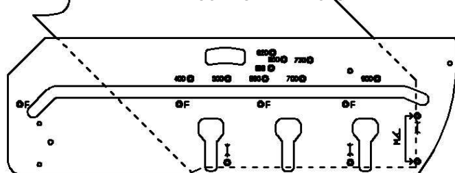
OBRÁZEK D DRÁŽKY PRO SVORNÍKY - SAMIČÍ SPOJ LÍCOVÁ STRANA DOLŮ
